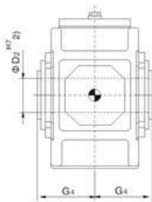
B3HH 空心轴
