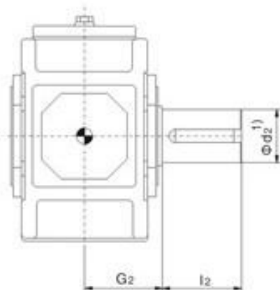
B4SH 实心轴
