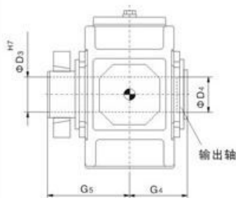
B4DH 带胀紧盘的空心轴
