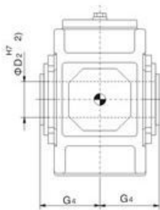
B4HH 空心轴
