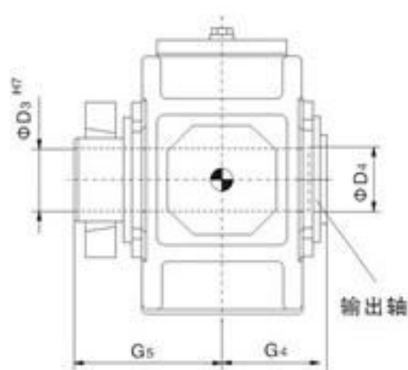
B3DH 带胀紧盘的空心轴
