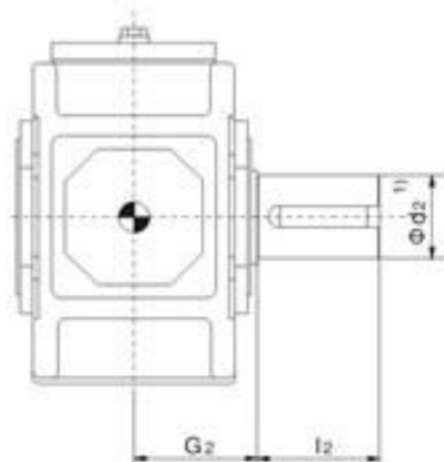
B3SH 实心轴
