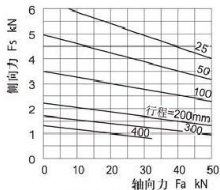
图6 SWL5(QWL5)
