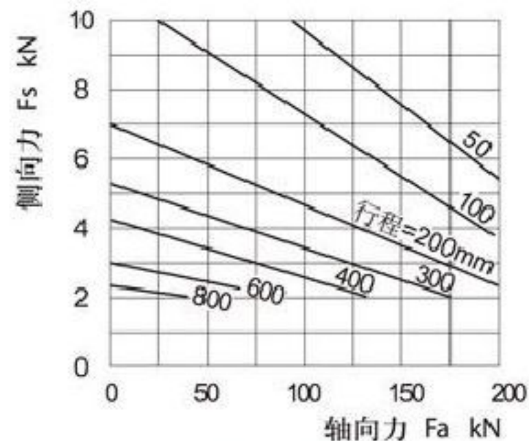
图8 SWL20(QWL20)
