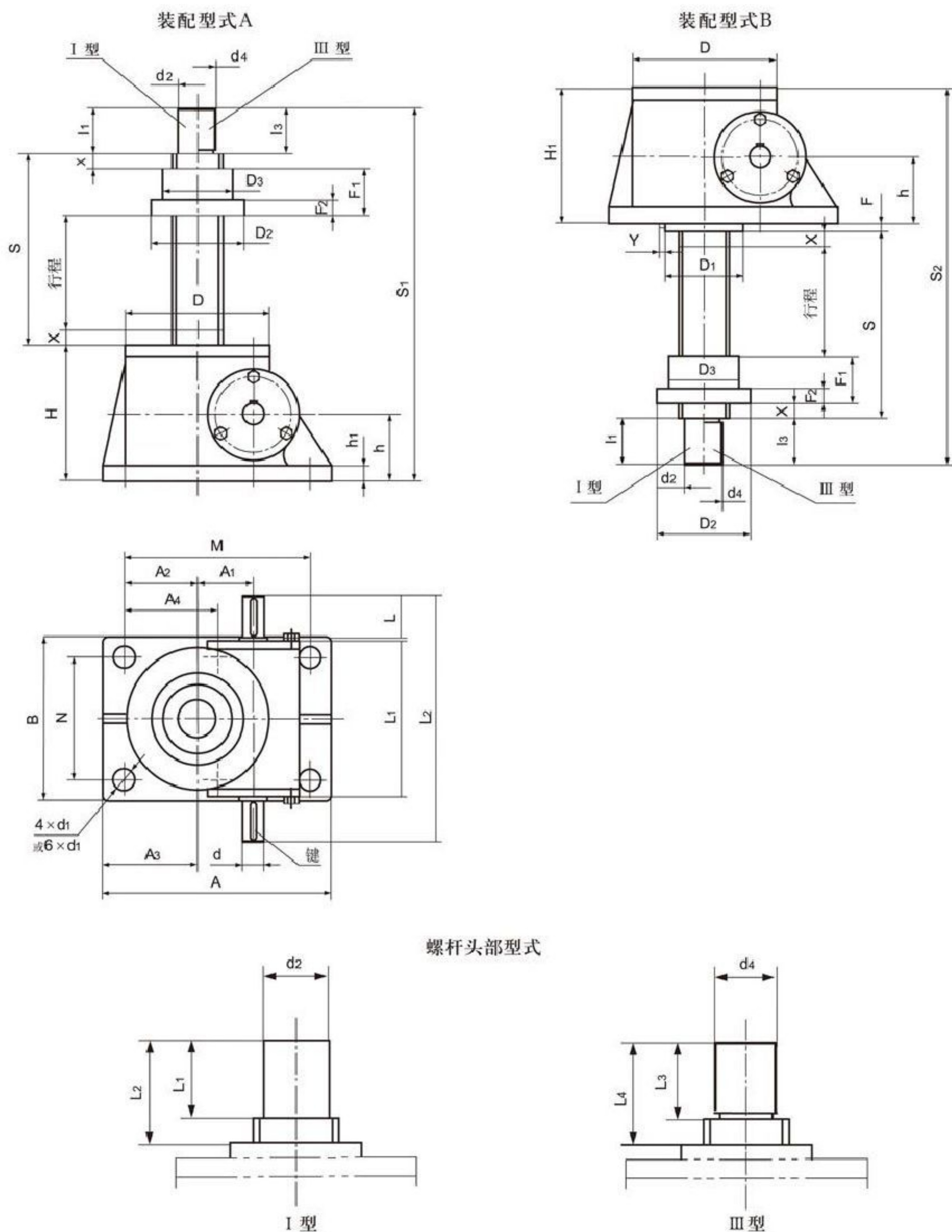
图2 2型结构型式
