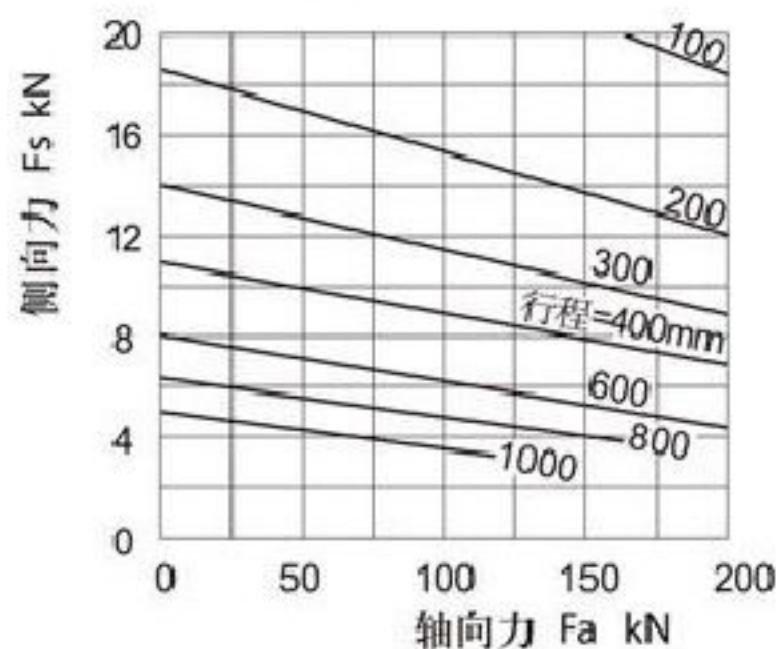
图9 SWL25(QWL25)
