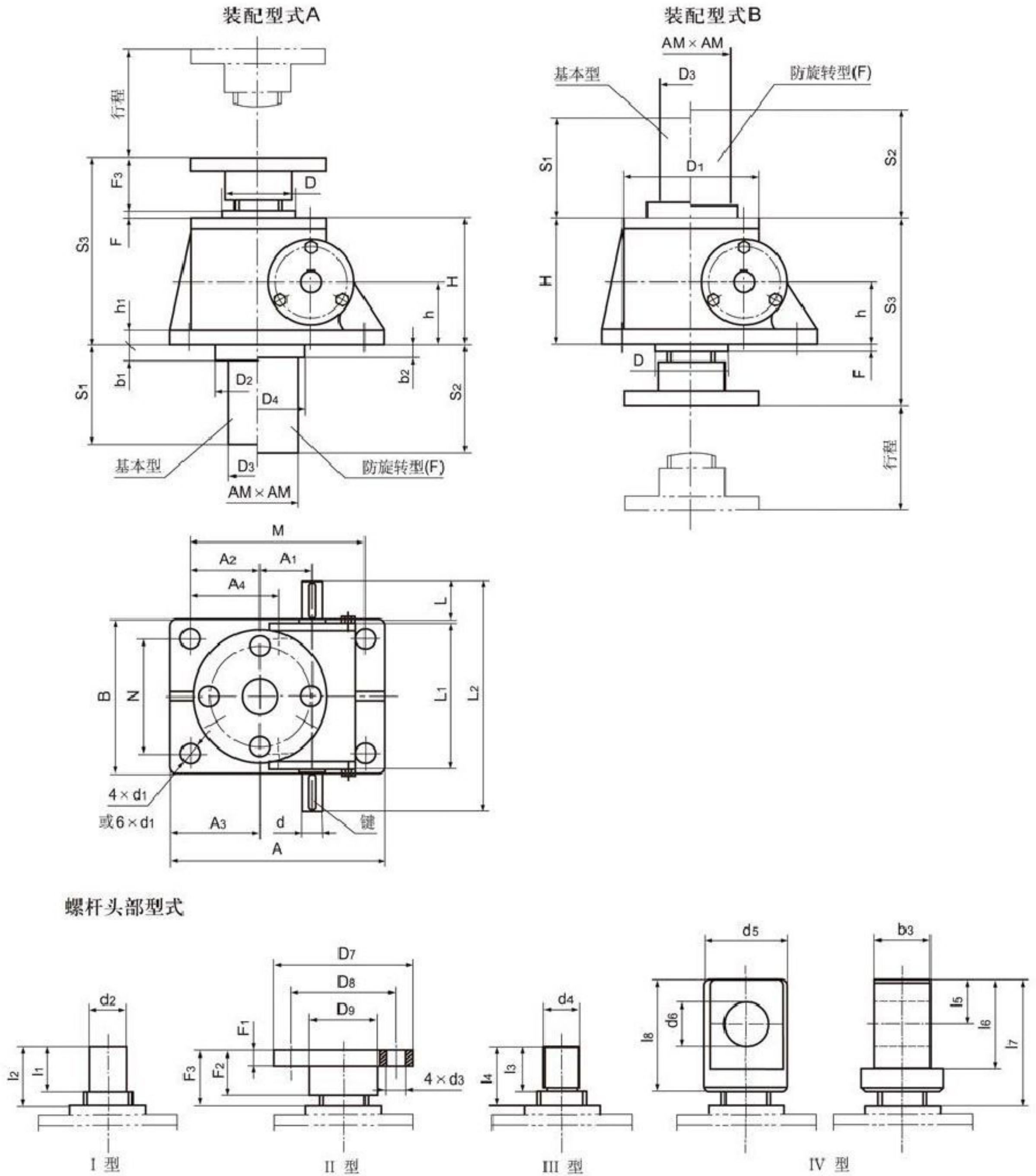
图1 1型结构形式
