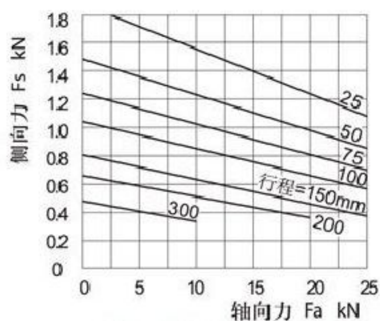
图5 SWL2.5(QWL2.5)
