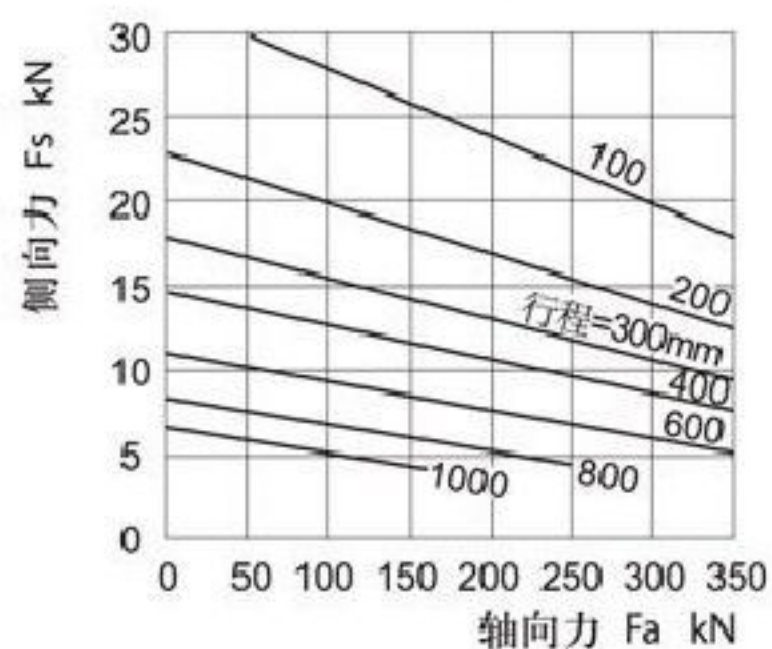
图10 SWL35
